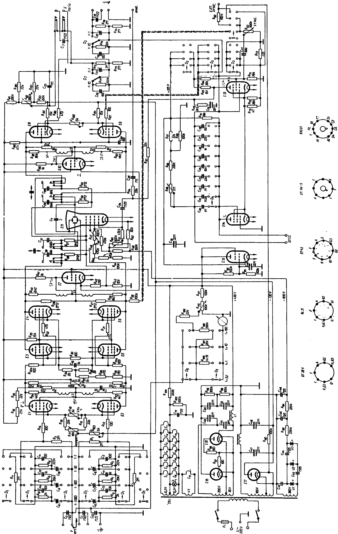
Schéma osciloscopu Křižák T 565
