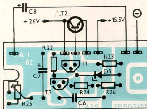
Deska stabilizátoru
