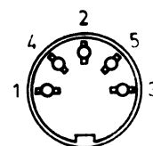
Obr. 3 Uspořádání dutinek pětipólové zásuvky při pohledu zvenku
