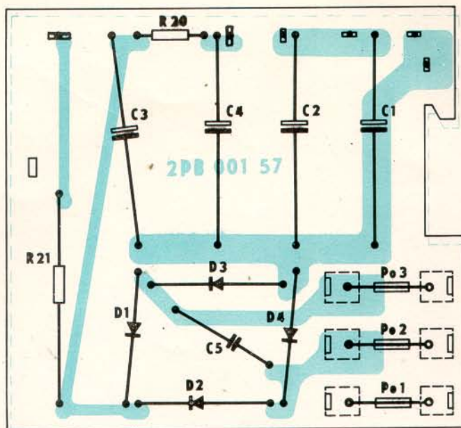
Deska napájení
