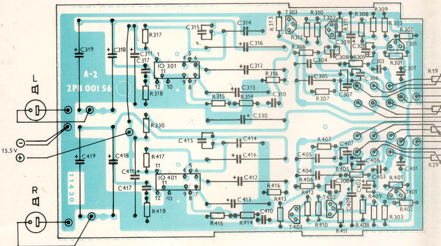
Deska výkonových zesilovačů
