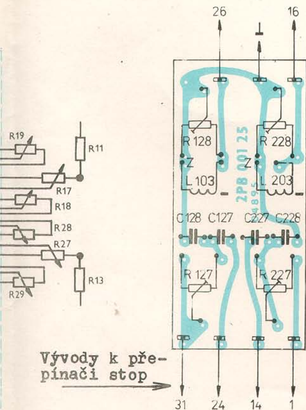
Deska trimrů
