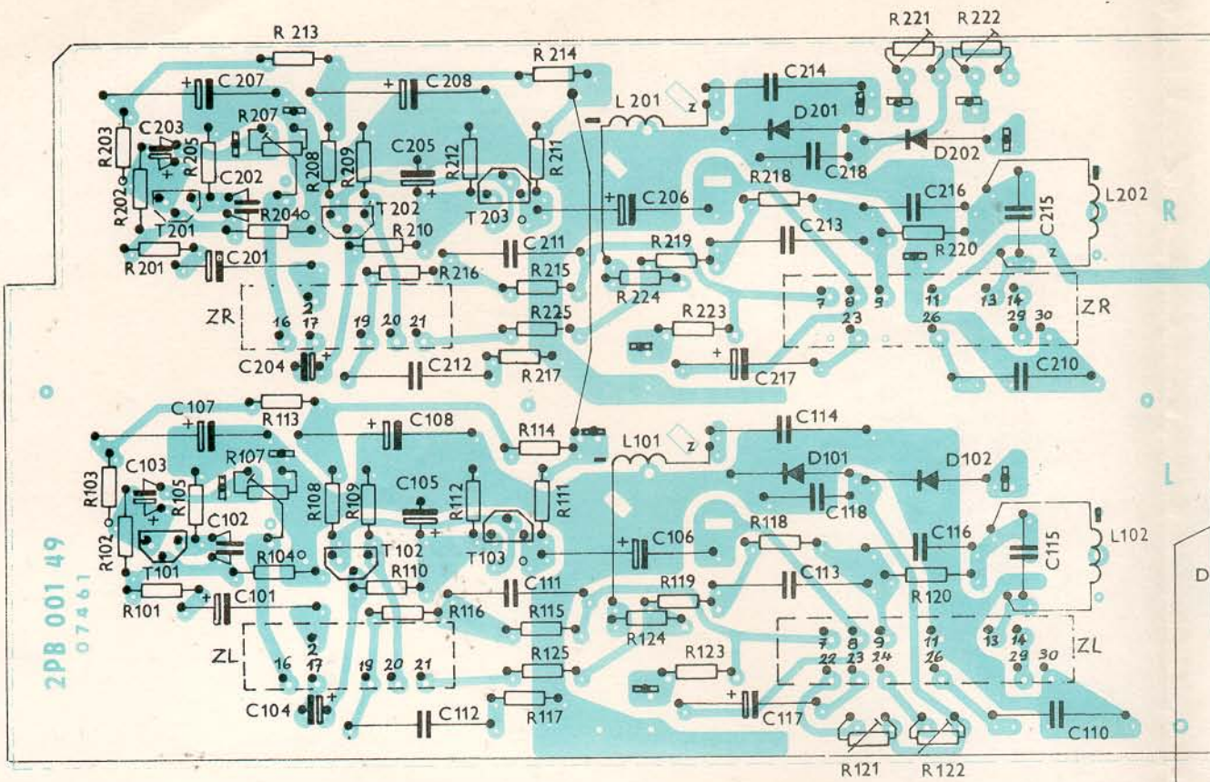
Deska snímacích/záznamových zesilovačů
