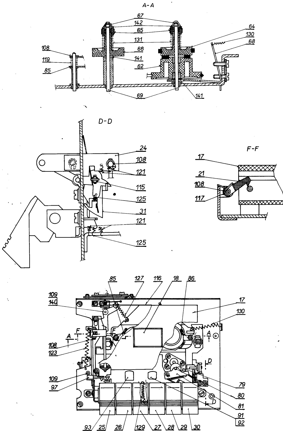
Pbr. 8. Náhradní díly - pohled shora
