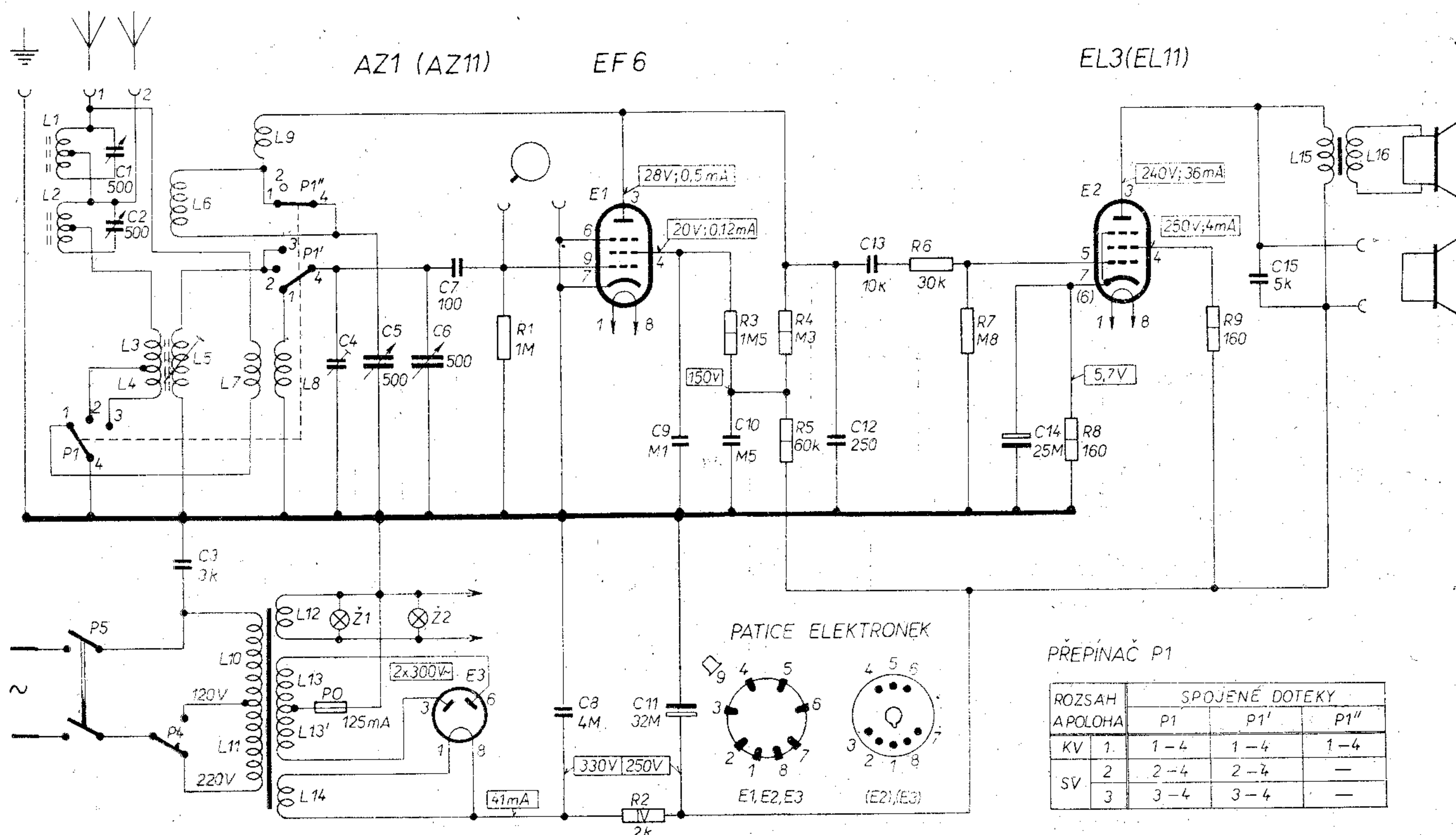
Zapojení přijímače SPEC IAL 47
